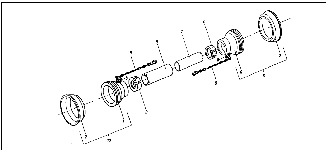
Rys. 31 ELEMENTY SKŁADOWE OSŁONY
