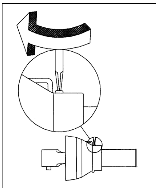
Rys. 26 WKRĘT MOCUJĄCY STOŻEK OSŁONY
