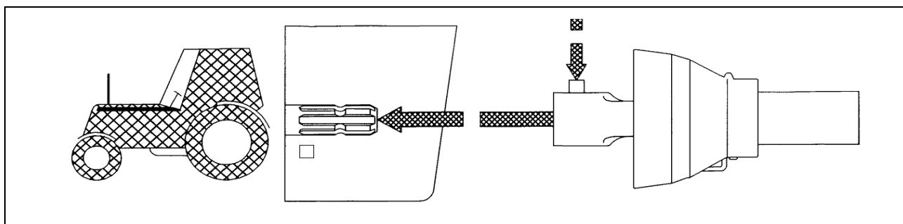
Rys. 8 AGREGOWANIE WAŁU NA WOM I WPM PRZY KONSTRUKCJI ZAPIĘCIA Z TRZPIENIEM ZATRZASKU
