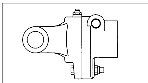
Rys. 29 SZKIC PRZEDSTAWIAJĄCY SPRZĘGŁO Z KOŁKIEM ŚCINANYM
