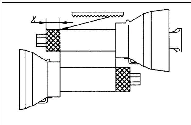
Rys. 12 SPOSÓB ODMIERZENIA ŻĄDANEJ DŁUGOŚCI I MIEJSCE ODCIĘCIA OSŁONY
