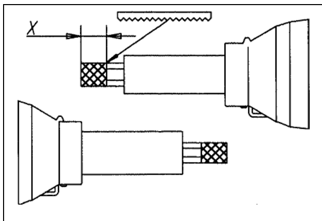
Rys. 13 SCHEMAT POKAZUJĄCY SPOSÓB SKRACANIA RUR TELESKOPU
