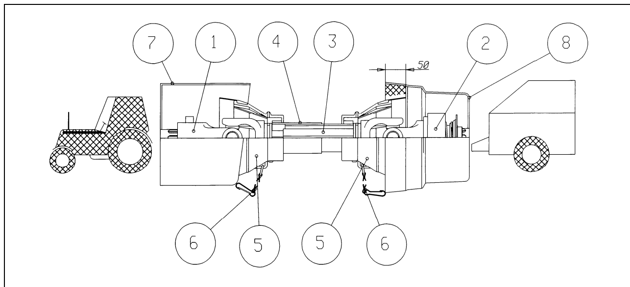
Rys. 4 SCHEMAT OGÓLNY PRZENIESIENIA NAPĘDU
