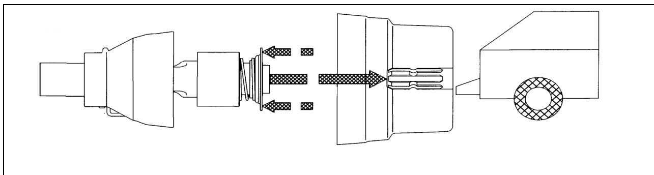
Rys. 9 AGREGOWANIE WAŁU NA WOM I WPM PRZY KONSTRUKCJI TRZYKULKOWEGO ZATRZASKU
