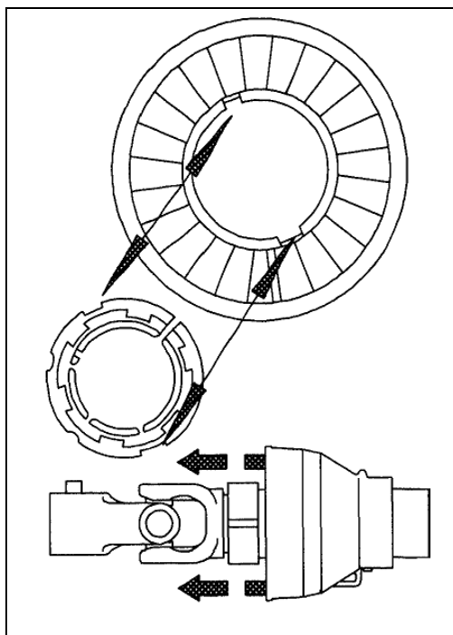
Rys. 24 NASUNIĘCIE STOŻKA OSŁONY NA RURĘ OSŁONY I PIERŚCIEŃ ŚLIZGOWY
