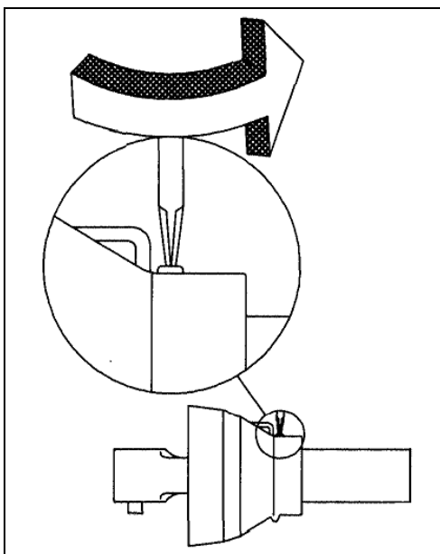
Rys. 17 WKRĘT MOCUJĄCY STOŻEK OSŁONY
