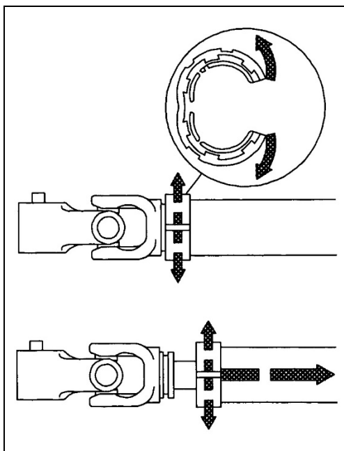
Rys. 20 ZSUNIĘCIE PIERŚCIENIA ŚLIZGOWEGO WRAZ Z RURĄ OSŁONY
