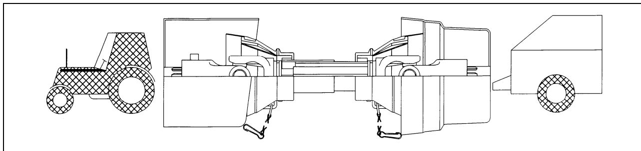
Rys. 1 PRZEZNACZENIE WAŁU PRZEGUBOWO-TELESKOPOWEGO
