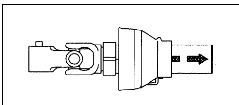
Rys. 19 ZSUNIĘCIE STOŻKA OSŁONY
