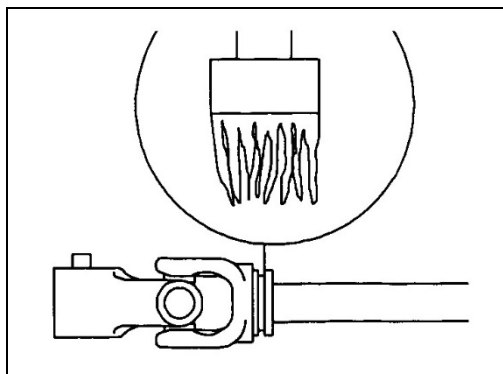
Rys. 22 SMAROWANIE KANAŁKA ŁOŻYSKOWEGO W WIDŁAKU
