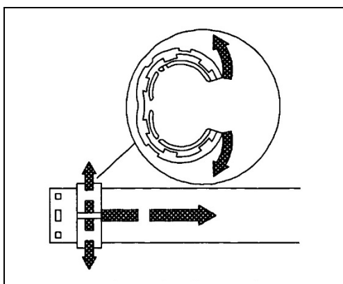
Rys. 21 ZSUNIĘCIE PIERŚCIENIA ŚLIZGOWEGO Z RURY OSŁONY
