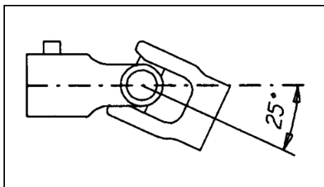
Rys. 6 DOPUSZCZALNY KĄT ŁAMANIA PRZEGUBU PRZY CIĄGŁEJ PRACY WAŁU
