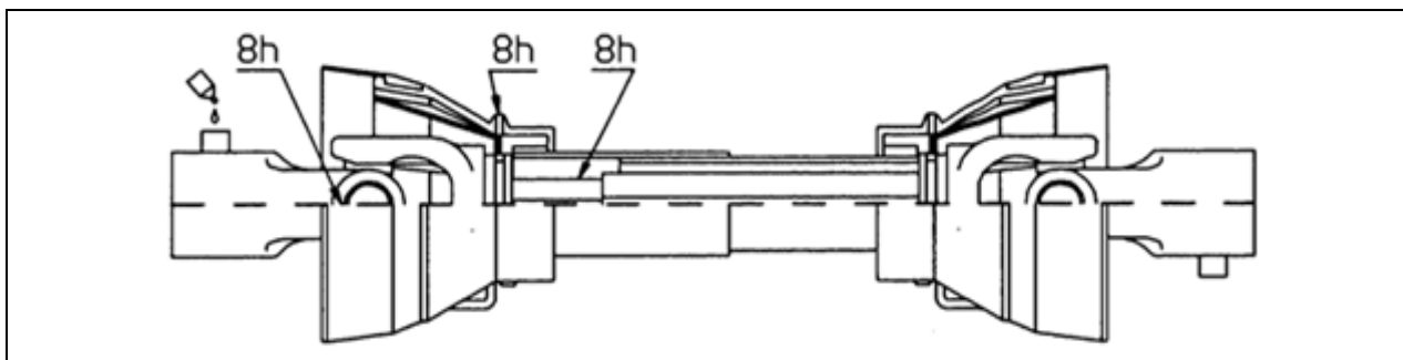
Rys. 11 SCHEMAT SMAROWANIA WAŁU PRZEGUBOWO-TELESKOPOWEGO
