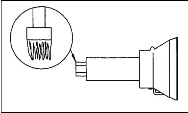
Rys. 15 SCHEMAT POKAZUJĄCY MIEJSCE SMAROWANIA RUR
