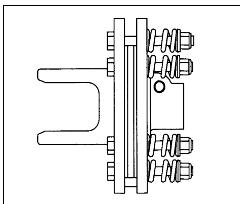
Rys. 28 SZKIC PRZEDSTAWIAJĄCY SPRZĘGŁO CIERNE
